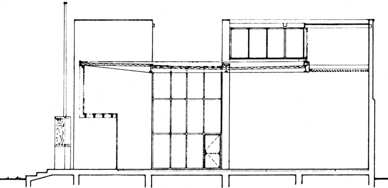
doorsnede A schaal 1:100
